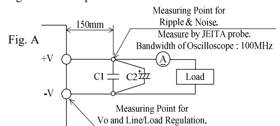
C1 : Film Cap. 0.1 μF C2 : Elec. Cap. 100 μF
