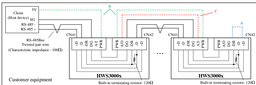
Figure 3-2 Actual wiring
