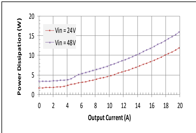
Vo = 9V
