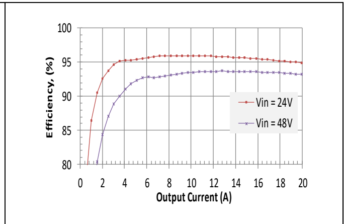
Vo = 12V
