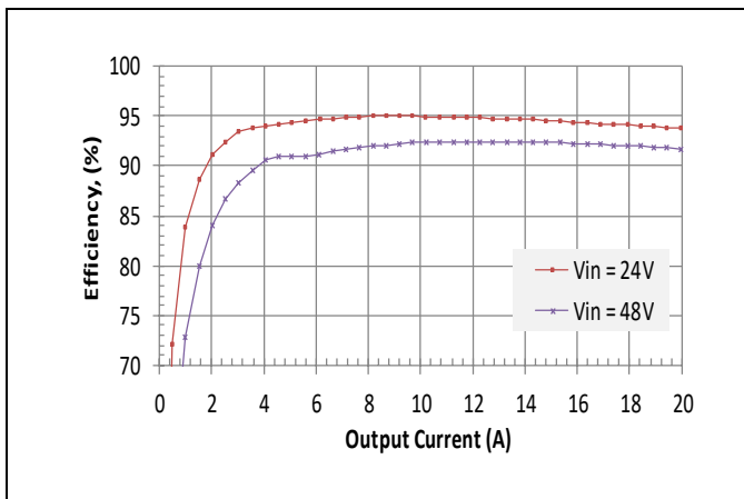
Vo = 9V
