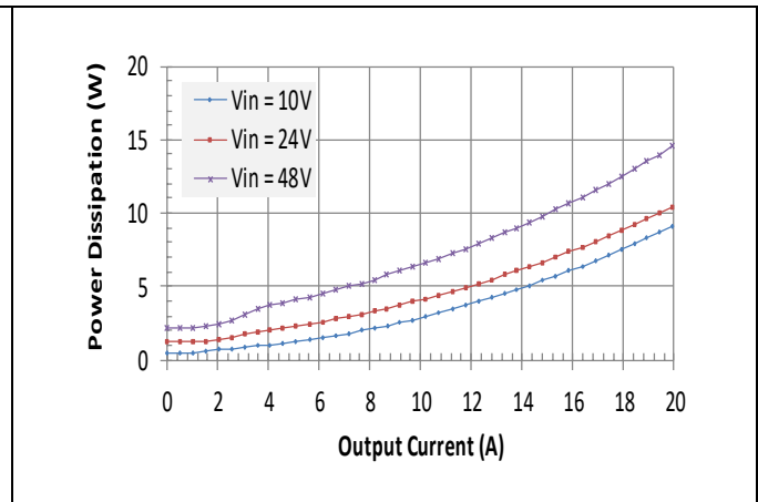
Vo = 5V
