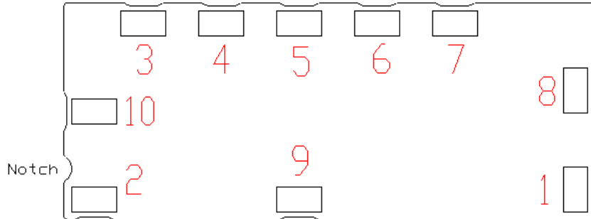
DOSA PINS
