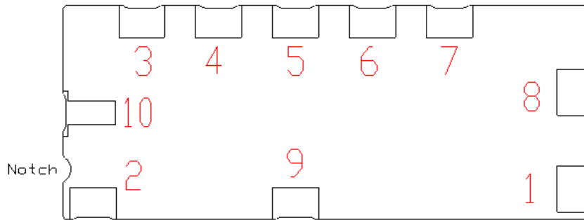
EPC PINS
