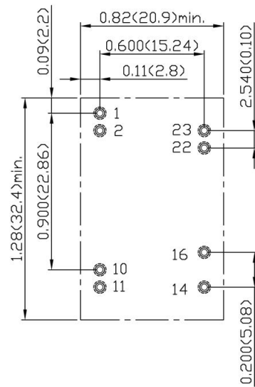
PXC-M03-xxWSxx B Type
