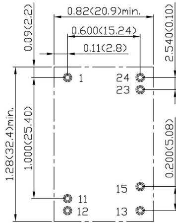
PXC-M03-xxWSxx A Type
