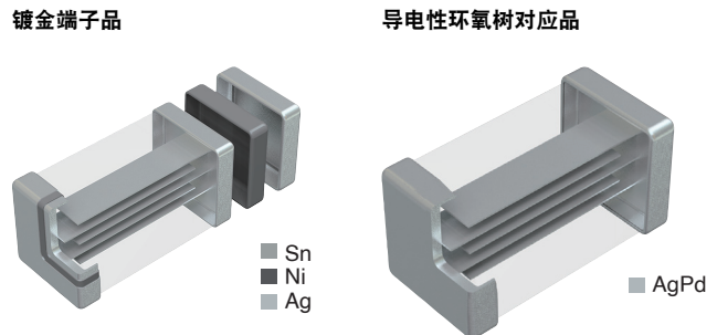
图2 积层贴片热敏电阻的内部结构
