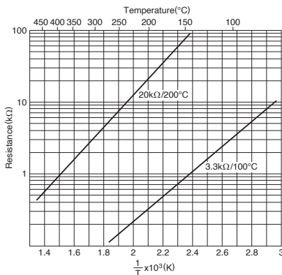
电阻 - 温度特性 (图1)
